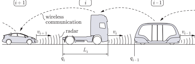
Fig. 1. CACC-equipped string of vehicles.
